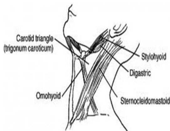
شکل ۱. نمای شماتیک از عضله کتفی لامی
