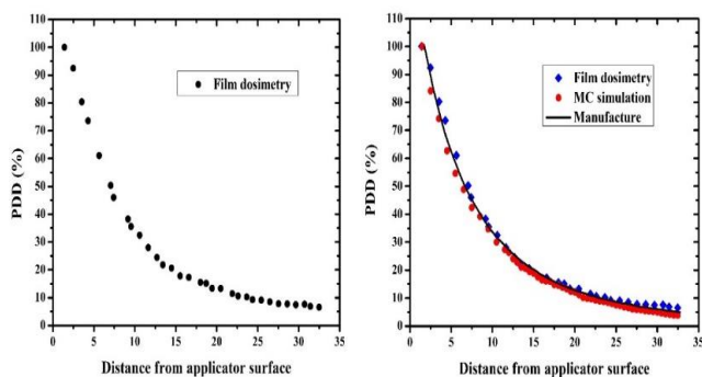
شکل ۸. منحنی PDD حاصل از فیلم دوزیمتری در اطراف اپلیکاتور ۲/۵ cm (چپ) و مقایسه نتایج با داده های بدست آمده توسط شبیه سازی مونت کارلو و مقادیر گزارش شده توسط سازنده (راست).
