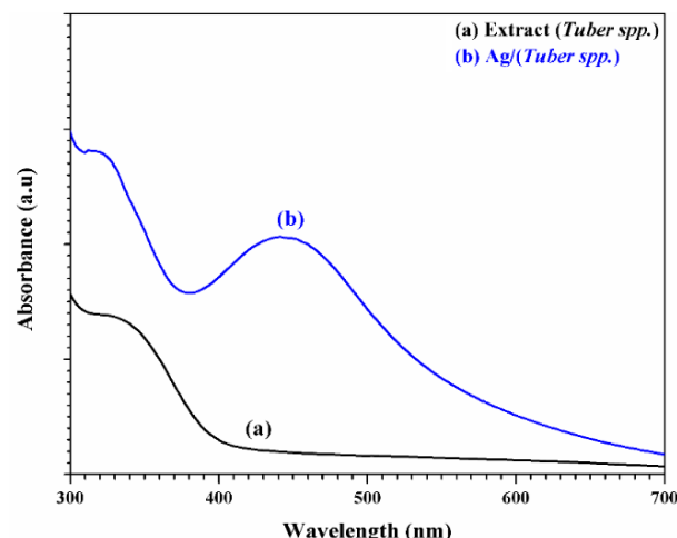
شکل ۱. جذب اسپکتروفتومتری (UV-Vis) عصاره، (a) نانوذرات نقره (b)
