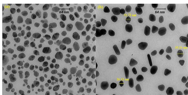
شکل ۴. (a, b) تصاویر TEM نانوذرات نقره سنتز شده از عصاره آبی ( Tuber spp. )
