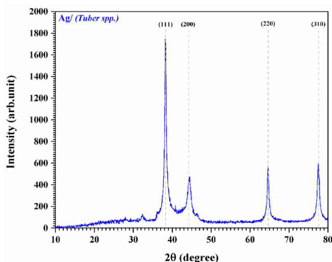
شکل ۲. الگوی پراش اشعه ایکس XRD از نانوذرات نقره سنتز شده در مدت زمان ۷۲ ساعت از عصاره قارچ دنبان ( Tuber spp. )
