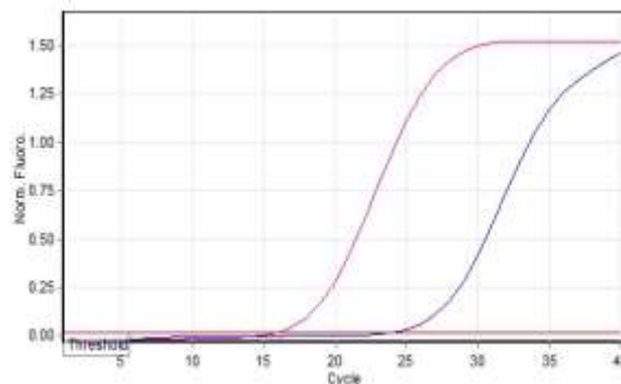
نمودار ۲. سیکل ترازد بیومارکرها- محور افقی شماره سیکل ترازد و محور عمودی میزان فلورسنت می باشد. مقدار CT برای ژن، EGFR ۲۴/۱۰ و برای ژن، FGFR4 ۱۶/۰۱ می باشد
