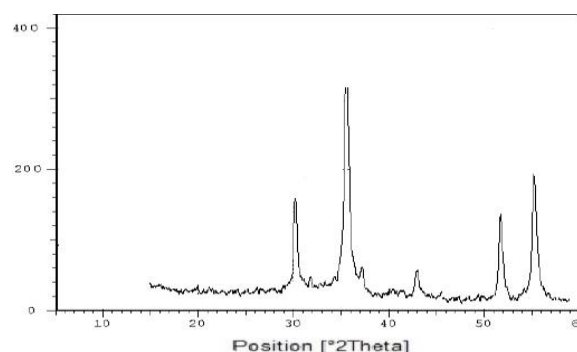
شکل ۲. الگوی XRD از نانو ذرات Fe 3 O 4
