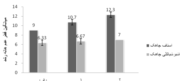
نمودار ۱. میانگین قطر عدم هاله رشد در غلظت‌های مختلف عصاره متانولی گیاه Ammimajus بر روی باکتری‌های استافیلوکوک اورئوس و اشریشیاکلی به روش چاهک
