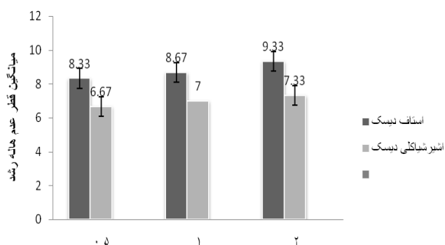
نمودار ۲. میانگین قطر عدم هاله رشد در غلظت‌های مختلف عصاره متانولی گیاه Ammimajus بر روی باکتری‌های استافیلوکوک اورئوس و اشریشیاکلی به روش دیسک
