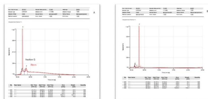
نمودار ۲. A: کروماتوگرام حاصل از تزریق فراکشن G به روش HPLC با زمان ماندگاری ۳:۳۹. B: کروماتوگرام حاصل از تزریق سارکوفین به روش HPLC
