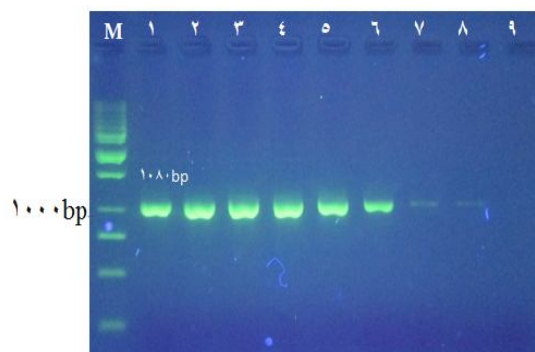
شکل 2. آزمون تعیین حد تشخیص PCR بهینه شده ژن TEM در باکتری کلبسیلا. SM: سایز مارکر فرمتاس 1kb DNA Ladder. 1. کنترل مثبت، 2. رقت 10^{-1} ، 3. رقت 10^{-2} ، 4. رقت 10^{-3} ، 5. رقت 10^{-4} ، 6. رقت 10^{-5} ، 7. رقت 10^{-6} ، 8. رقت 10^{-7} ، 9. کنترل منفی.
