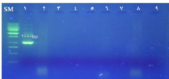
شکل 3. آزمون اختصاصیت PCR بهینه شده. SM. سایز مارکر شرکت فرمتاس 1kb DNA Ladder. 1. نمونه کنترل مثبت (DNA کلبسیلائی واجد ژن TEM)، 2. DNA کلبسیلائی فاقد ژن TEM، 3. DNA سالمونلا، 4. DNA مایکوباکتریوم توبرکلوزیس، 5. DNA مایکوپلاسما پنومونیه، 6. DNA کاندیدا آلبیکنس، 7. DNA بروسلا، 8. DNA اشیریشیا کلی فاقد ژن TEM، 9. کنترل منفی
