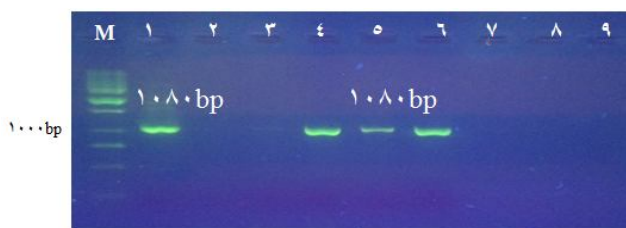
شکل 4. آزمون بهینه شده PCR تشخیص ژن TEM در کلبسیلا. SM: سایز مارکر فرمتاس 1Kb DNA Ladder. 1. کنترل مثبت با DNA کلبسیلائی واجد ژن TEM (1080 bp)، 2. 3، 4، 5، 6، 7، 8، 9. نمونه های منفی، 9. کنترل منفی
