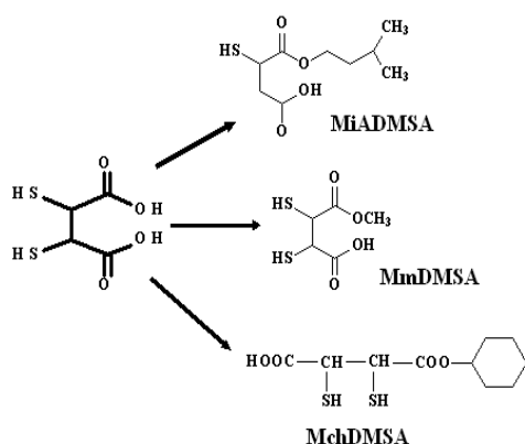
شکل ۵. مونواستر های جدید دی مرکاپتوسوسکسینیک اسید (DMSA)
