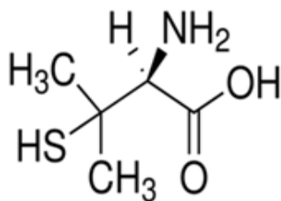
شکل ۲. D-Penicillamine (DPA)
