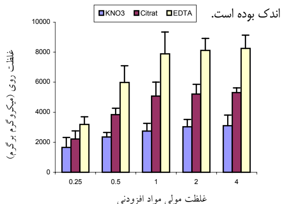
نمودار ۱. میزان فلز روی استخراجی بر حسب میکروگرم بر گرم خاک نمونه در غلظت های مختلف مواد افزودنی
