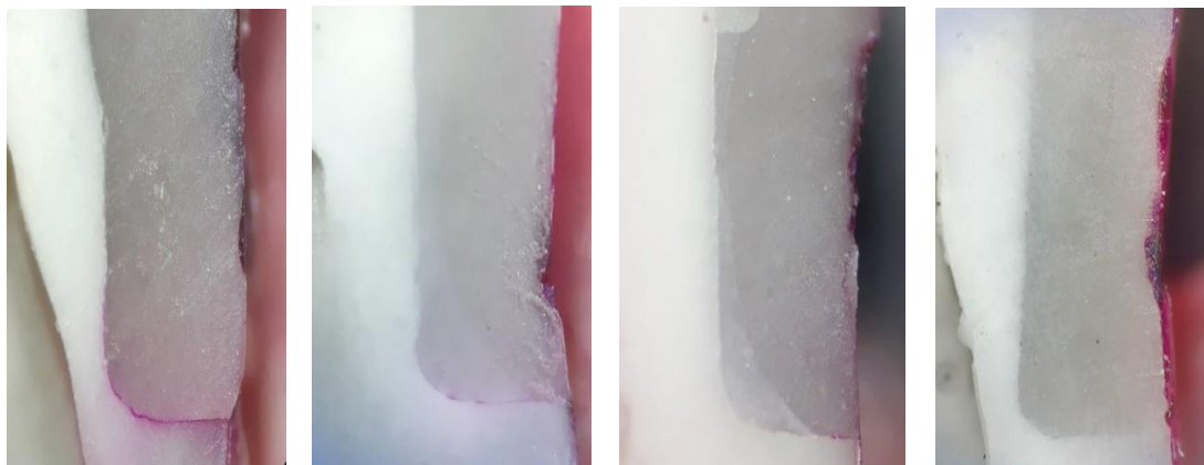
شکل ۱. ریزش رتبه صفر شکل ۲. ریزش رتبه ۱ شکل ۳. ریزش رتبه ۲ شکل ۴. ریزش رتبه ۳
