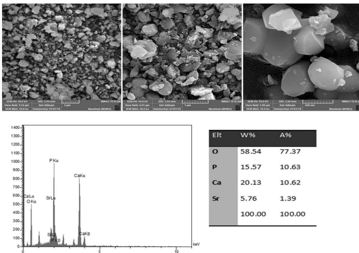
شکل ۴. تصویر SEM و آنالیز EDS ذرات استرنسیوم هیدروکسی آپاتیت
