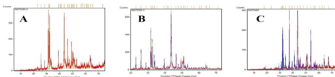
شکل ۱. الگوی XRD مربوط به سیلیسیوم هیدروکسی آپاتیت (A)؛ استرنسیوم هیدروکسی آپاتیت (B) و تری کلسیم سیلیکات (C)
