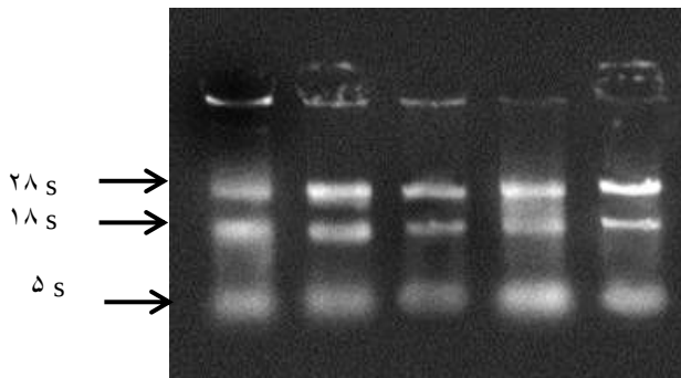
شکل ۳. نتیجه الکتروفورز پنج نمونه RNA استخراج شده از گروه‌های مختلف آزمایشی. در ژل آگارز ۱٪ وجود سه باند واضح (rRNA 18s, rRNA 28s, و rRNA 5s) در ژل آگارز نشان دهنده صحت فرآیند تخلیص و عدم تخریب نمونه‌های RNA می‌باشد
