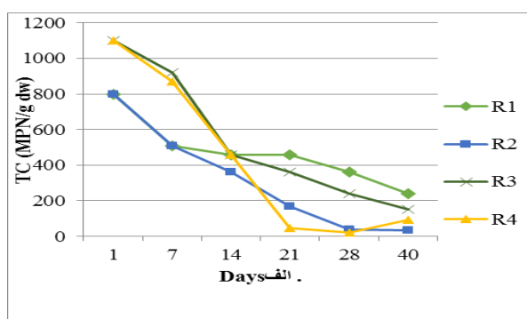
نمودار ۶. درصد تغییرات (الف) توتال کلیرم و (ب) فیکال کلیرم در طی فرایند کمپوست و ورمی کمپوست در چهار راکتور R1, R2, R3 و R4
