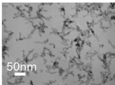
شکل ۱. تصویر میکروسکوپ الکترونی گذاره (TEM) نانوذرات اکسیدمس
