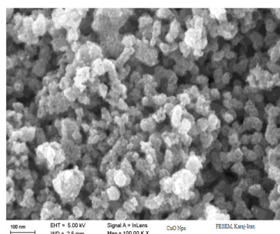
شکل ۲. تصویر لایه های نانوذرات اکسیدمس در میکروسکوپ الکترونی روبشی (SEM)
