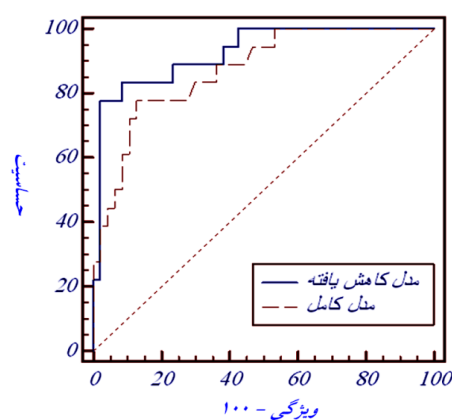
شکل ۴: مقایسه منحنی ROC مدل کامل و مدل کاهش یافته.
