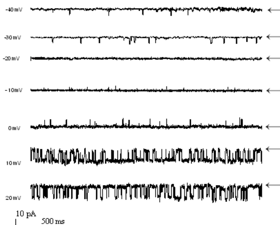
شکل ۳: ثبت از فعالیت کانال پتاسیمی پس از اضافه نمودن غلظت ۵۰ میلی مولار \text{Na}_2\text{HPO}_4 به محیط ترانس در ولتاژهای مختلف و در محیط (۲۰۰ mM KCl cis/۵۰ mM KCl trans).
