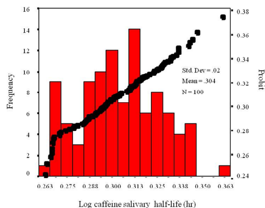
نمودار ۱. توزیع فراوانی و probit plot (منحنی احتمال) نیمه عمر کافئین با در نظر گرفتن کل جامعه شرکت کننده در مطالعه تعیین فنوتایپ آنزیم CYP1A2 در داوطلبین سالم مازندران
