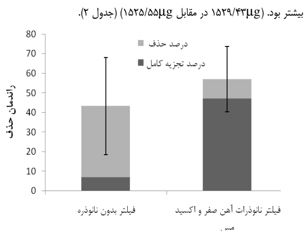
نمودار ۱. میانگین و انحراف معیار راندمان حذف و درصد تجزیه کامل ترکیبات BTX در فیلتر بدون نانوذره و فیلتر حاوی نانوذرات آهن و اکسید مس
