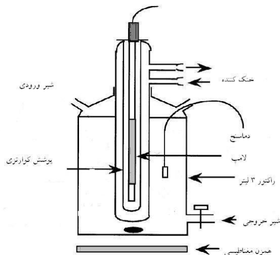
شکل ۳. اجزای شماتیک رآکتور فرابنفش
