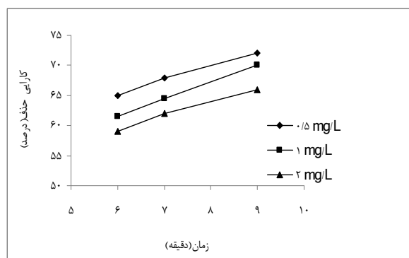
نمودار ۱. کارایی حذف مالاتیون بوسیله پرتوهای فرابنفش در غلظت های مختلف
