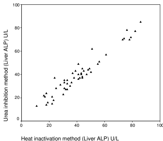
نمودار ۱. همبستگی بین نتایج روشهای غیرفعال سازی حرارتی و مهار با اوره در اندازه گیری فعالیت ایزوآنزیم کبدی آلکالین فسفاتاز سرم ( r=0/964 )
