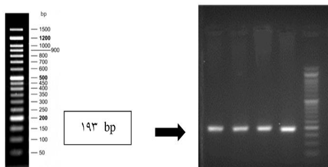
شکل ۱. الکتروفورز ژل آگارز ۲٪ برای تعدادی از محصول PCR افراد بیمار و مارکر ۵۰ جفت‌باز. (نقشه مارکر اندازه مولکول در این شکل آورده شده است)
